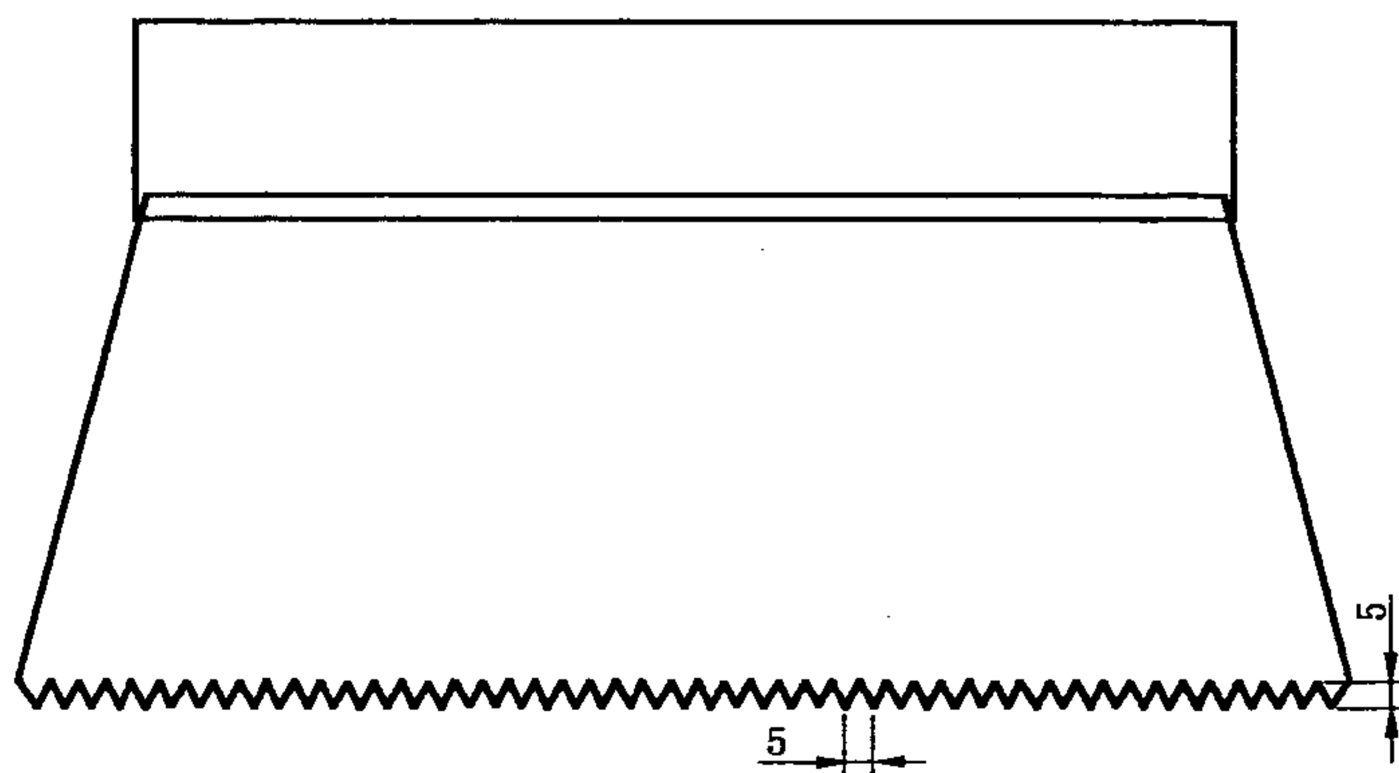
图 1 梳齿刮刀
